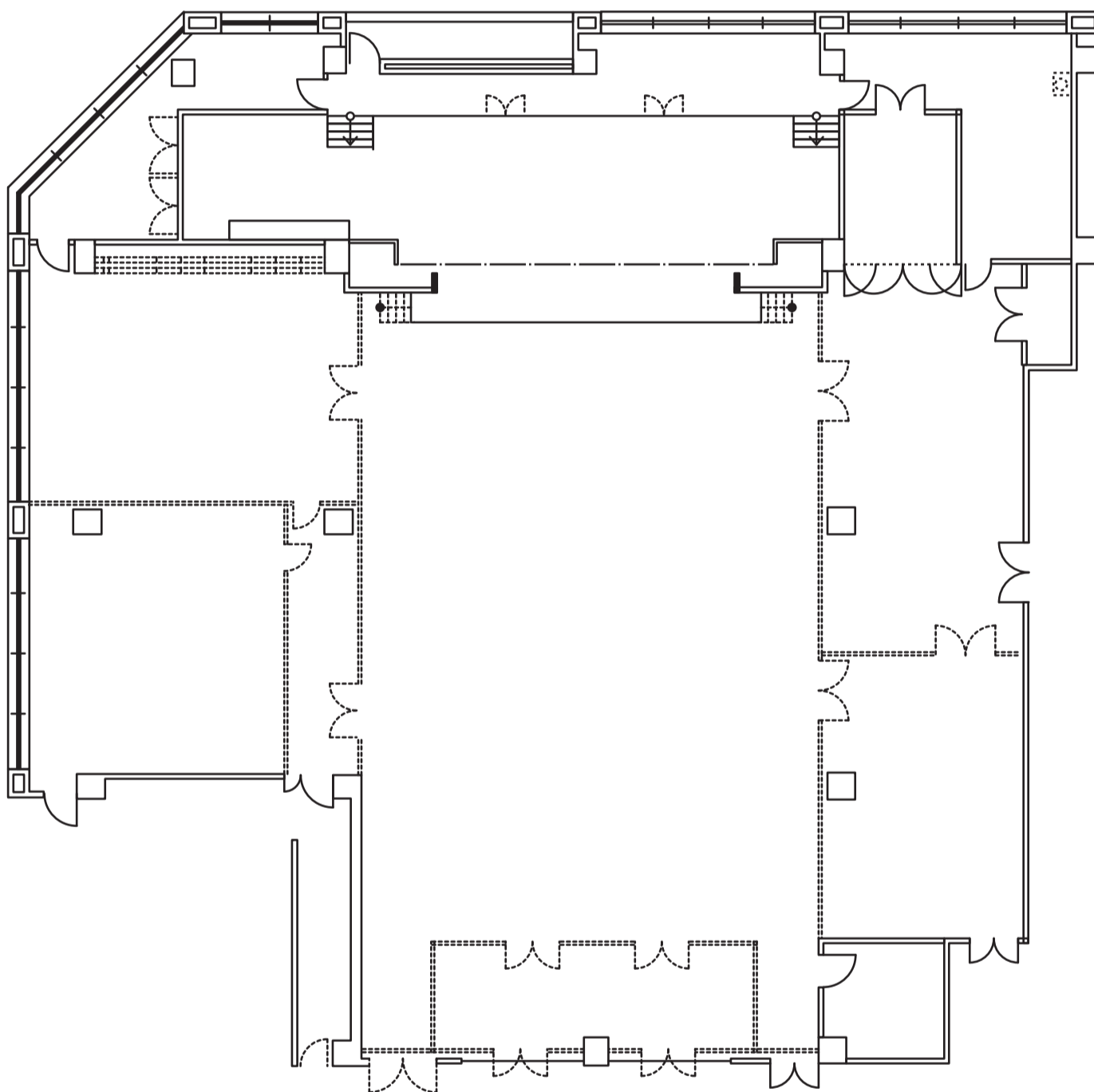
平面图 1/200
